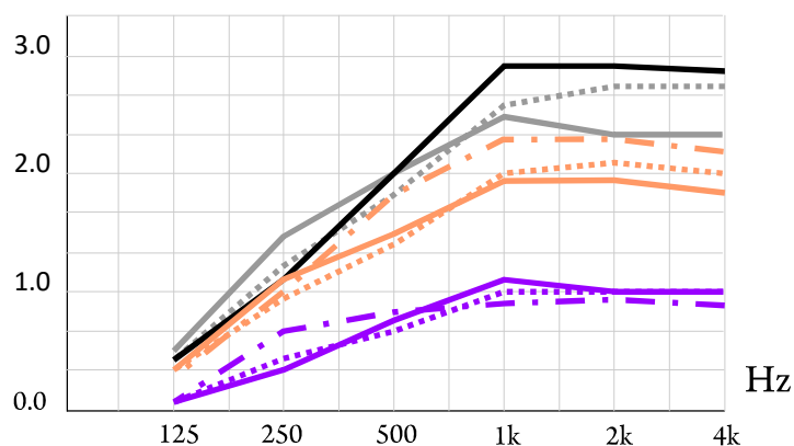
Эквивалентная площадь звукопоглощения, м 2 /панель
